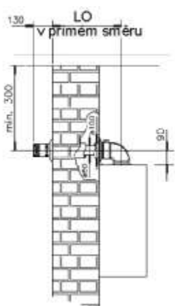
systém horizontálního odtahu spalin
