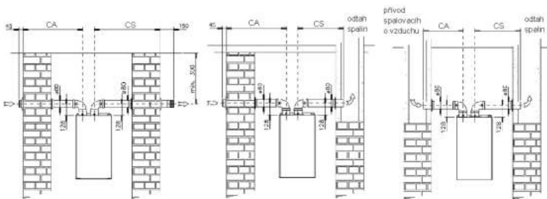
rozdvojený odtah spalin a přívod spalovacího vzduchu
