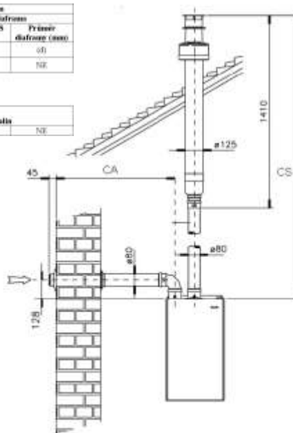
přívod spalovacího vzduchu z prostoru a odtah spalin pomocí komína nad střechu
