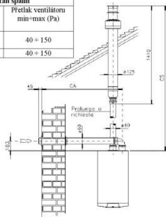
odtah spalin do komína přes střechu a přívod spal. vzduchu z venkovního prostředí
