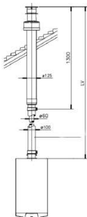
sousý odtah spalin přes střechu
