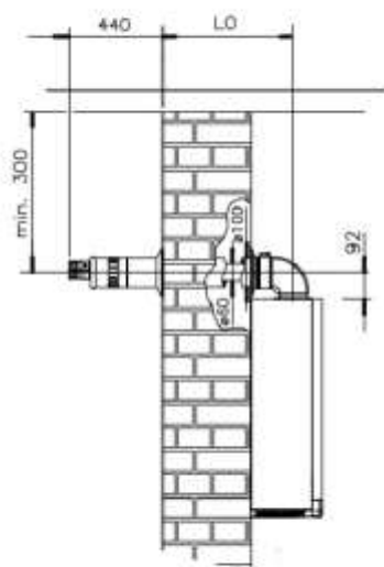
sousý odtah spalin přes obvodové zdivo
